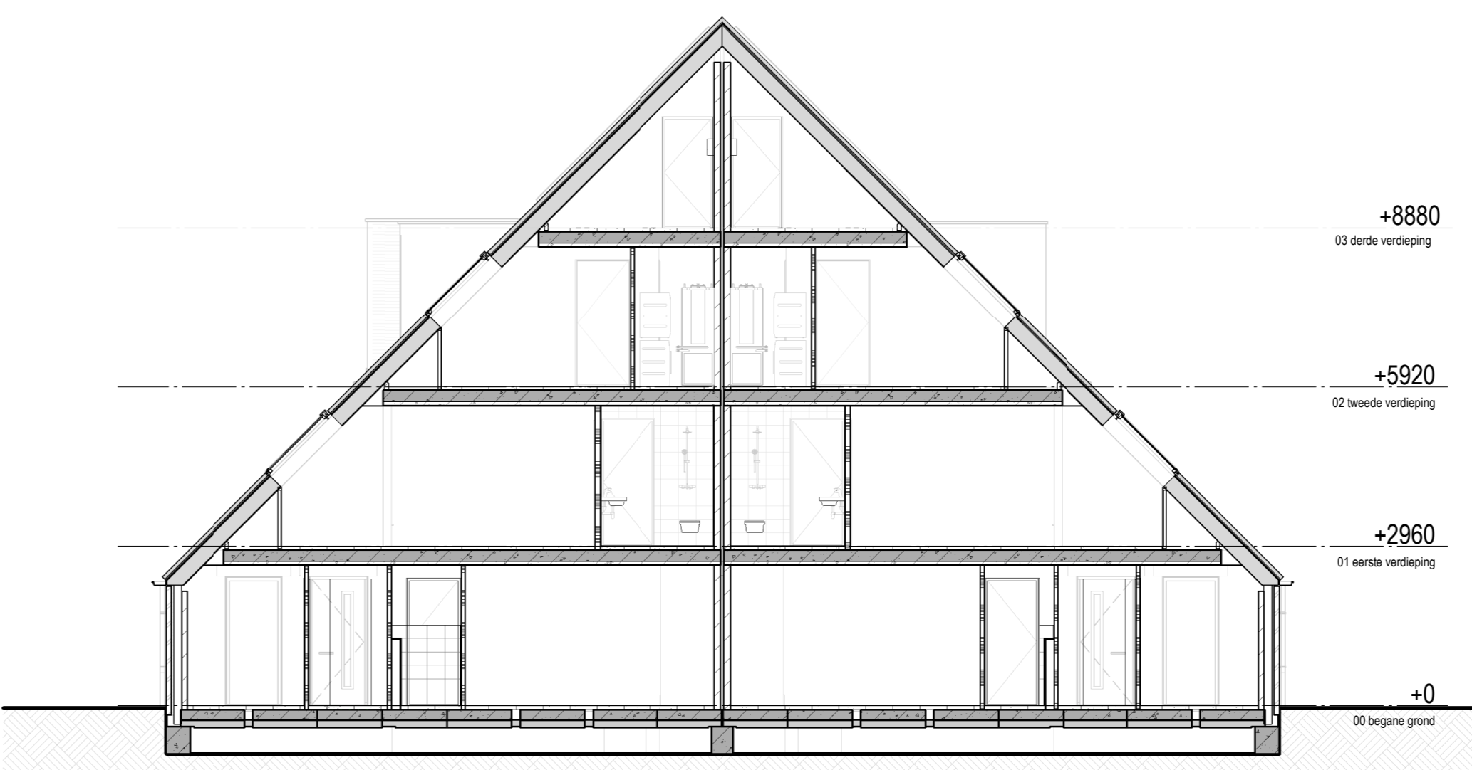
Doorsnede KK2 1:100
