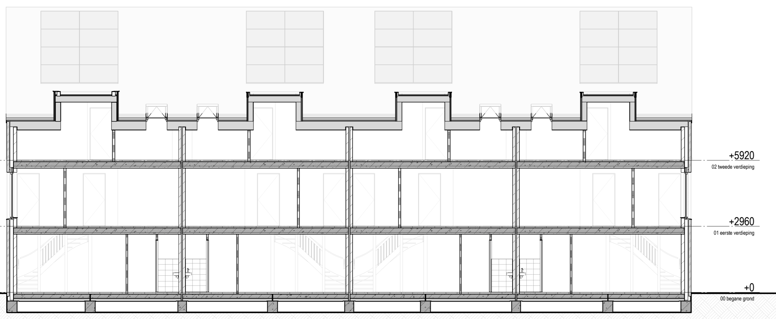
Doorsnede KK1 1:100
