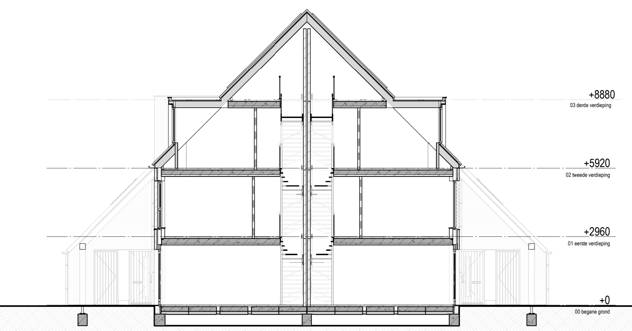
Doorsnede KK3 1:100
