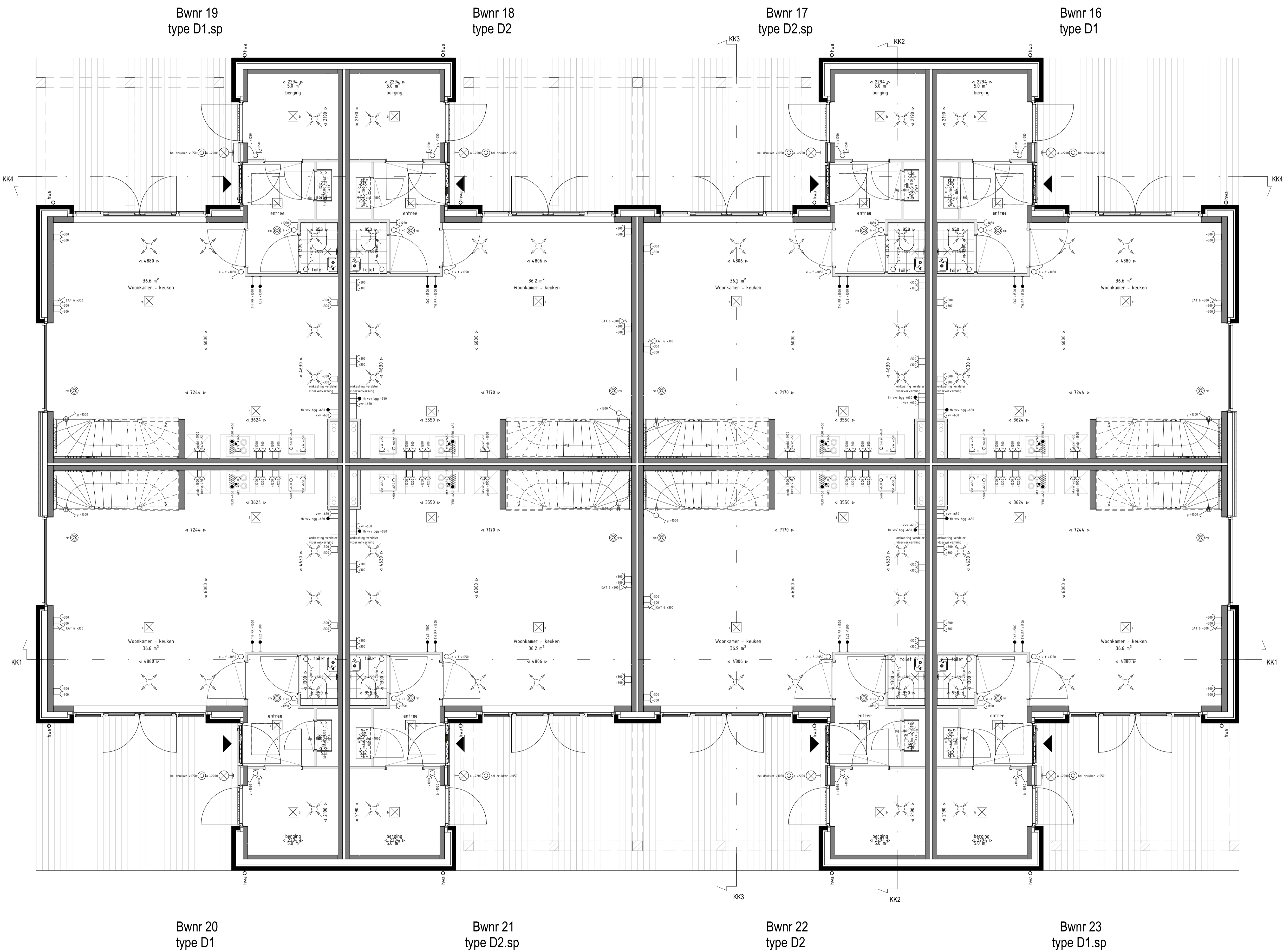
Begane grond 1:50
