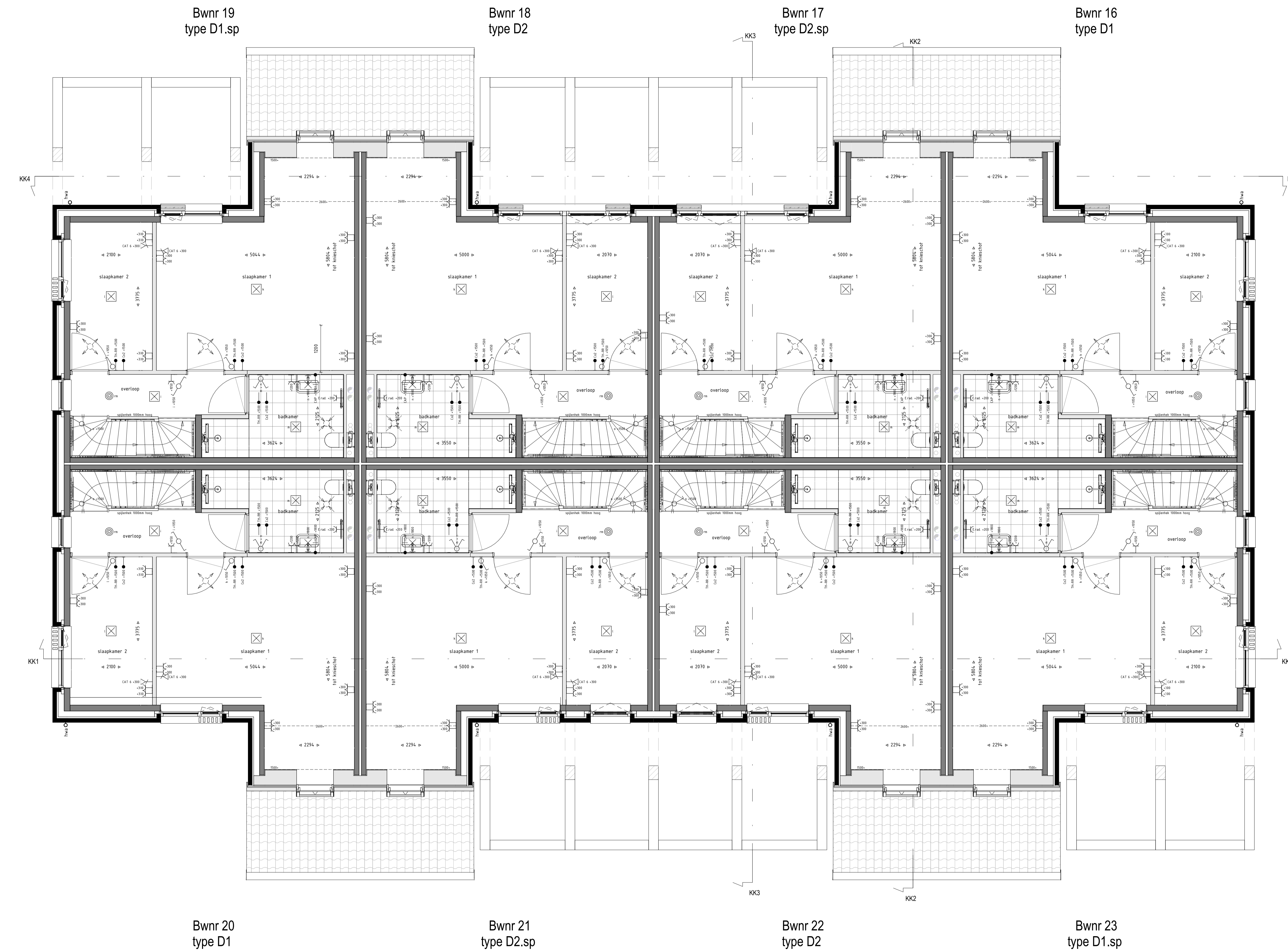
Eerste verdieping 1:50
