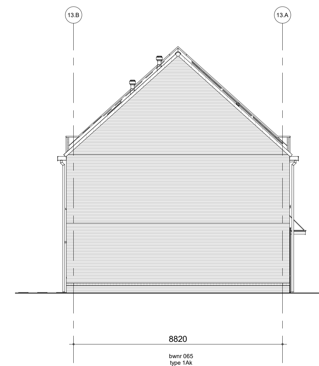
zijgevel links - blok 13
