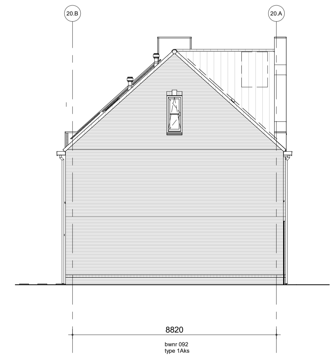
zijgevel links - blok 20
