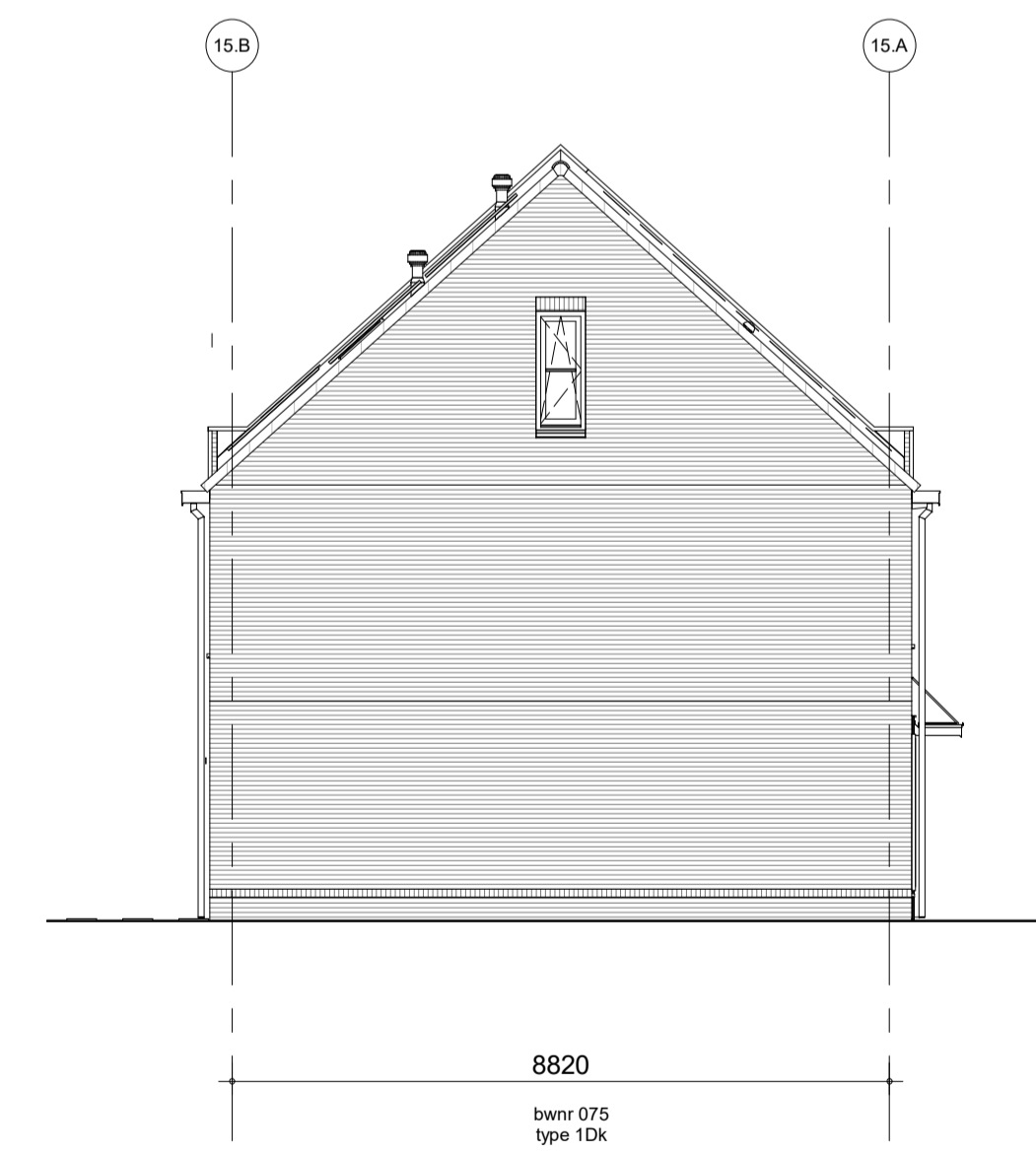
zijgevel links - blok 15
