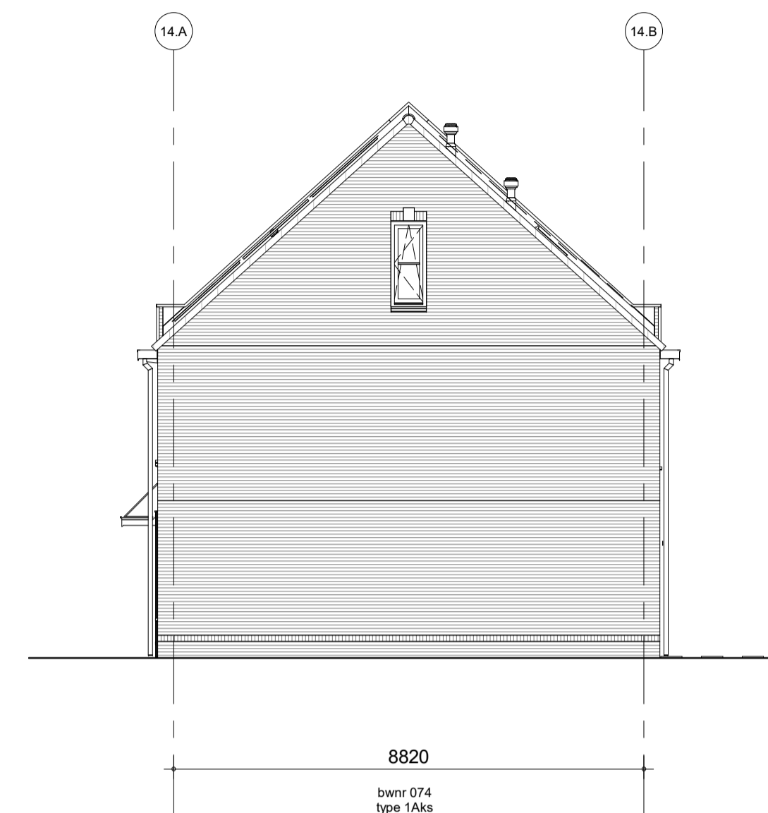
zijgevel rechts - blok 14
