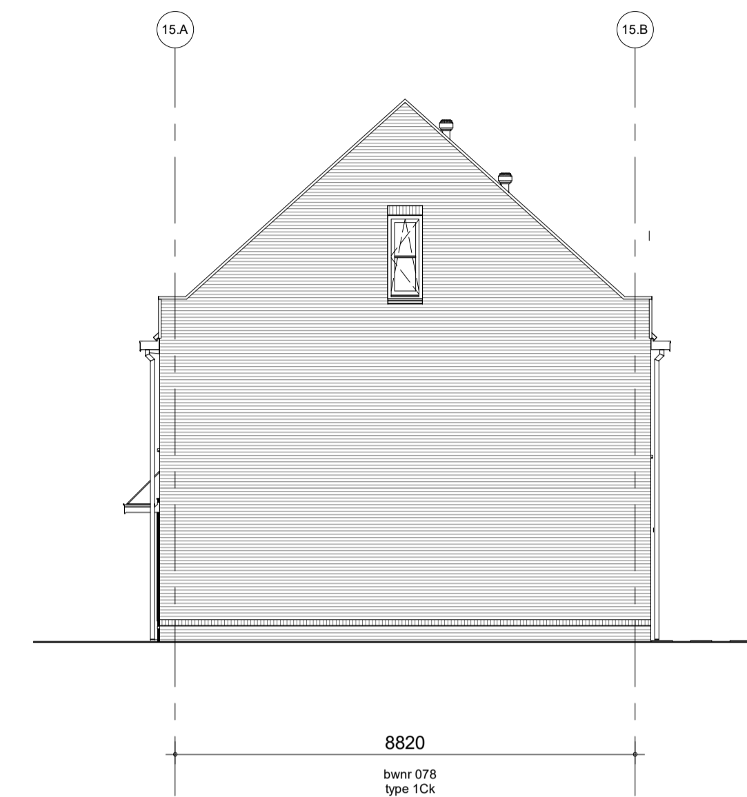
zijgevel rechts - blok 15
