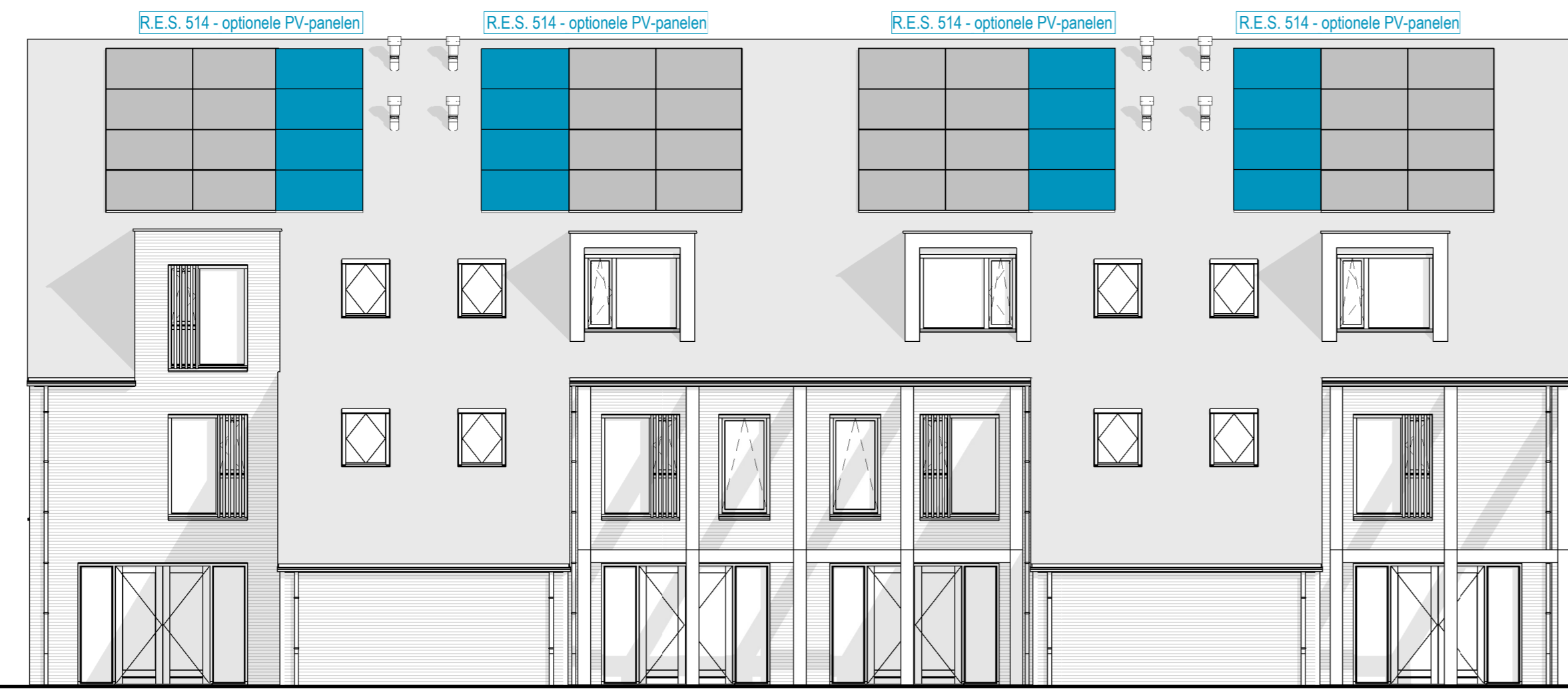
Zuidoost gevel - PV panelen 1 : 100
